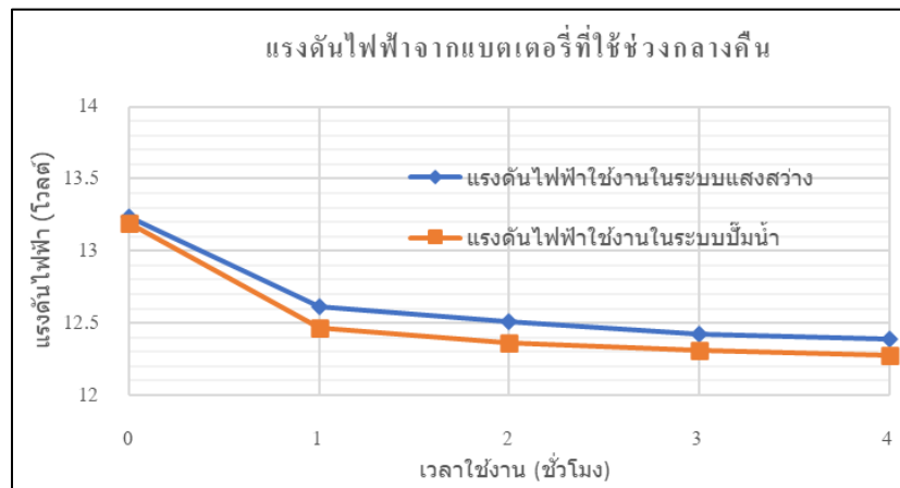
รูปที่ 8 กราฟทดลองใช้พลังงานจากแบตเตอรี่เมื่อโซลาร์เซลล์หยุดชาร์จ
