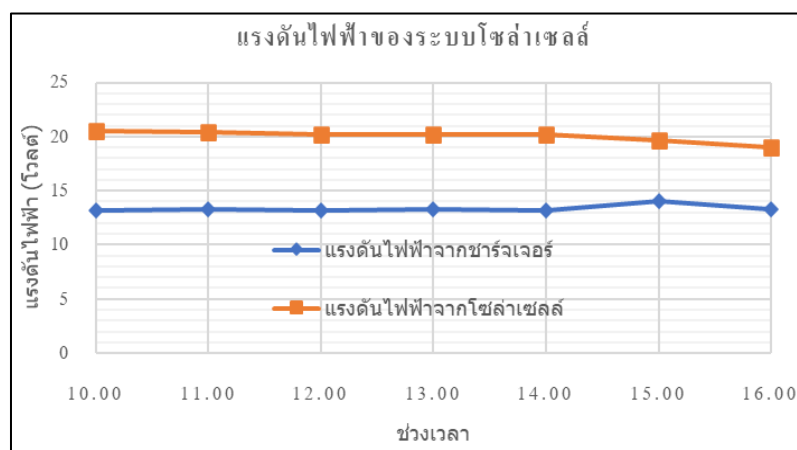
รูปที่ 6 แรงดันไฟฟ้าของระบบโซลาร์เซลล์
