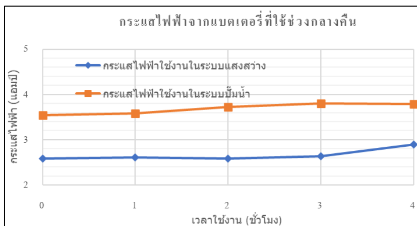
รูปที่ 9 กระแสไฟฟ้าของโหลดจากแบตเตอรี่เมื่อโซลาร์เซลล์หยุดชาร์จ
