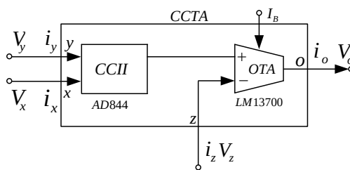
รูปที่ 2 โครงสร้างภายในของ CCTA
