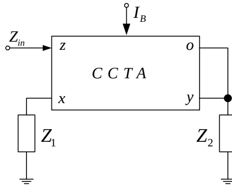
รูปที่ 3 วงจรเสมือนอุปกรณ์แบบต่อลงกราวด์ที่นำเสนอสอน
