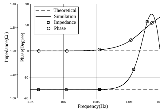
รูปที่ 4 อิมพีแดนซ์และเฟสเมื่อวงจรทำหน้าที่เป็นตัวต้านทาน
