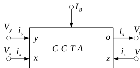
รูปที่ 1 สัญลักษณ์ของวงจรขยายความนำถ่ายโอนสายพานกระแส
