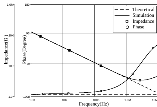
รูปที่ 6 อิมพีแดนซ์และเฟสเมื่อวงจรทำหน้าที่เป็นตัวเก็บประจุ
