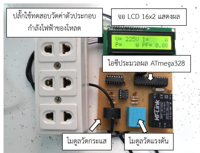
รูปที่ 4 ลักษณะโครงสร้างอุปกรณ์จริงของวงจรวัดค่าตัวประกอบกำลังไฟฟ้า
