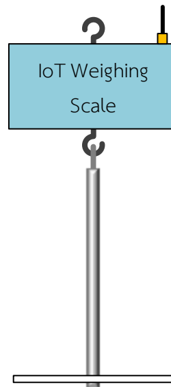
รูปที่ 3 แบบของต้นแบบเครื่องชั่งน้ำหนักแบบประสาบบอินเทอร์เน็ตของสรรพสิ่ง
