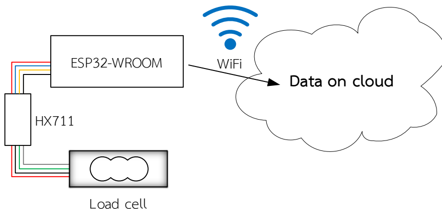
รูปที่ 2 ระบบโครงสร้างอุปกรณ์ของต้นแบบเครื่องชั่งน้ำหนัก ทำงานร่วมกับระบบอินเตอร์เน็ตประสานสรรพสิ่ง
